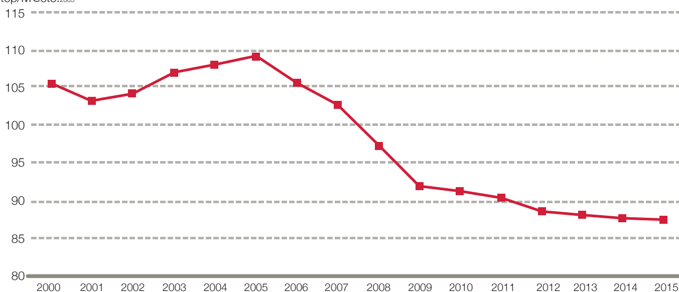
Figura 34. Evolución, la intensidad energética primaria en el periodo 2000-2015.
